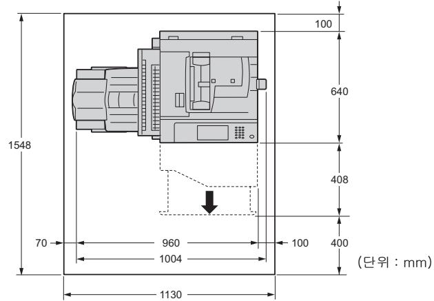
자동양면원고이송장치와 측면 트레이 (옵션) 가 장착된 경우
