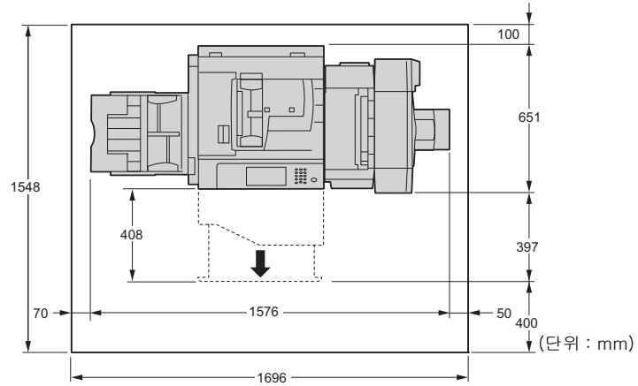
B1 Finisher 용 Booklet 유니트 (옵션) 가 장착된 경우
