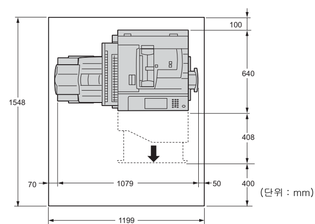
A1 Finisher (옵션) 와 측면 트레이 (옵션) 가 장착된 경우
