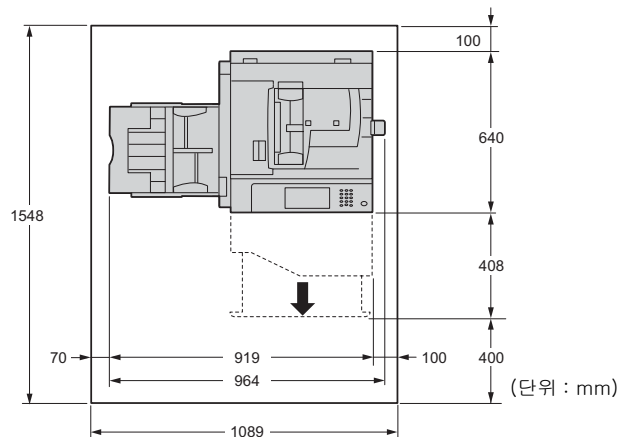
자동양면원고이송장치가 장착된 경우
