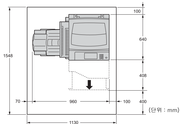
자동양면원고이송장치가 장착된 경우
