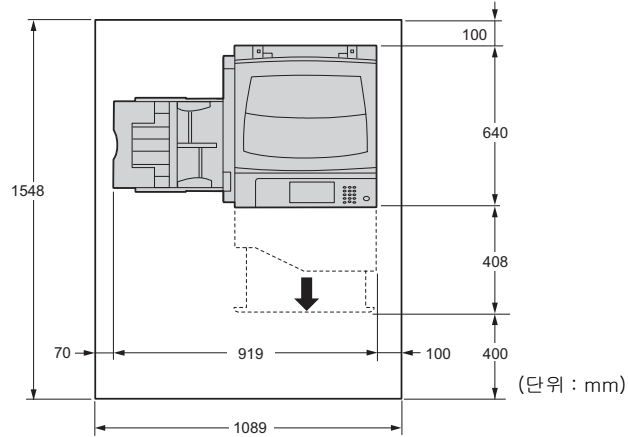
원고대 커버가 장착된 경우
