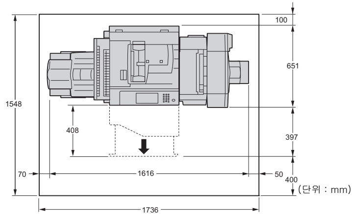
B1 Finisher 용 Booklet 유니트 (옵션) 와 측면 트레이 (옵션) 가 장착된 경우
