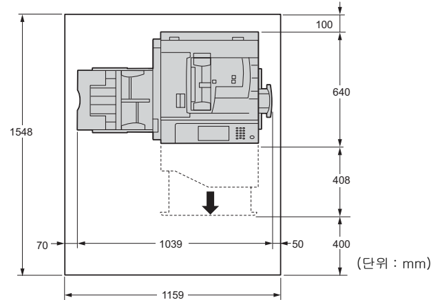
A1 Finisher (옵션) 가 장착된 경우
