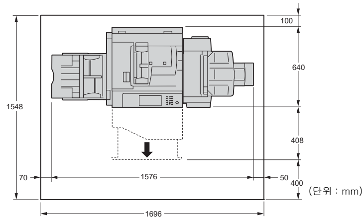
B1 Finisher (옵션) 가 장착된 경우
