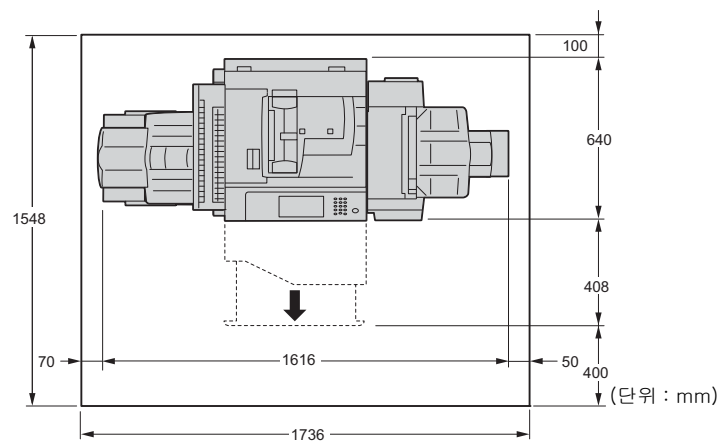
B1 Finisher (옵션) 와 측면 트레이 (옵션) 가 장착된 경우
